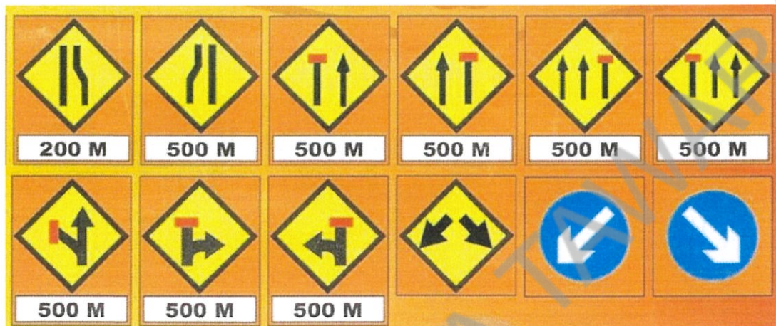
1.1 Papan tanda amaran/makluman sementara
