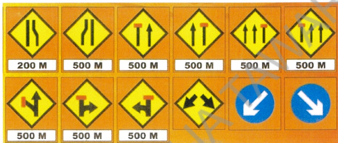
1.1 Papan tanda amaran/makluman sementara
