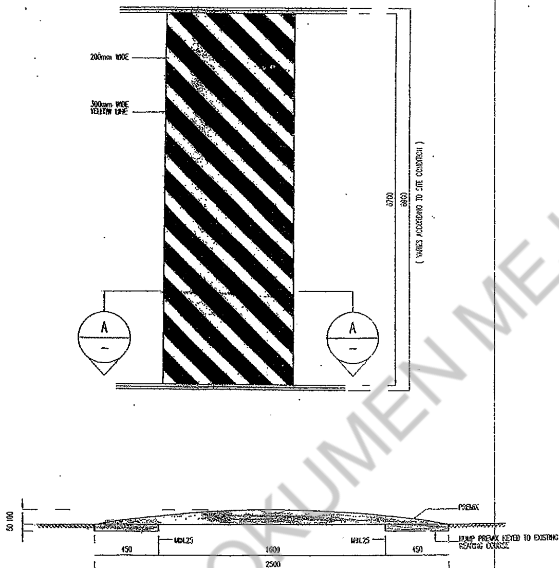
SECTION A-A
