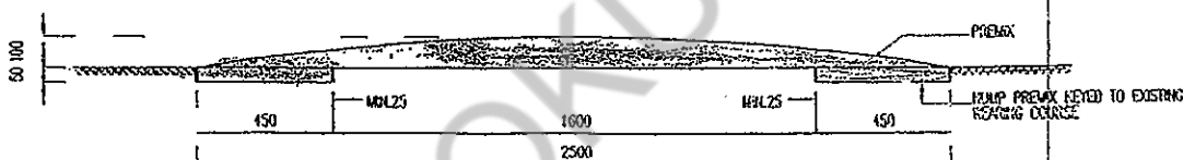
SECTION A-A
